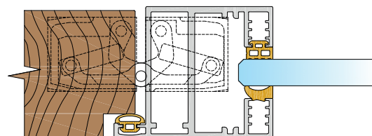
Dřevěné | zárubeň P10 | Tectus TE 340 | až 37 dB
