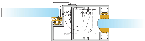
Celoskleněné | zárubeň P09 | Tectus TEG 310 | až 32 dB
