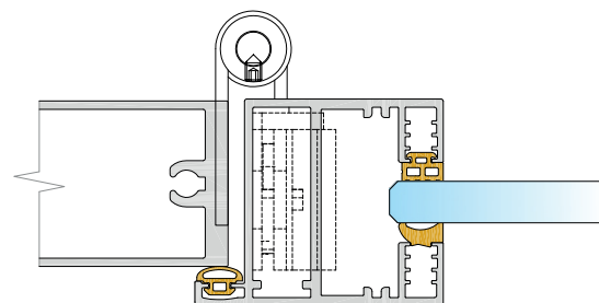
Hliníkové | zárubeň P10 | Just 3D | až 37 dB
