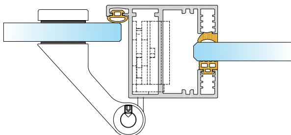
Celoskleněné | zárubeň P10 | Just 3D | až 32 dB
